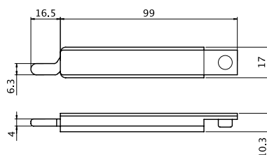
Terminale asta R40 punta piatta
