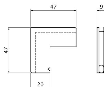
Squadretta gola asimmetrica
