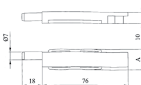
Terminale asta R40 Ø 7
