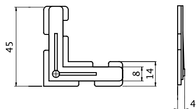
Squadretta Allineamento R40
