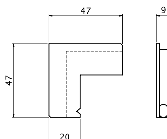
Squadretta gola simmetrica
