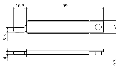
Terminale asta R40 punta piatta
